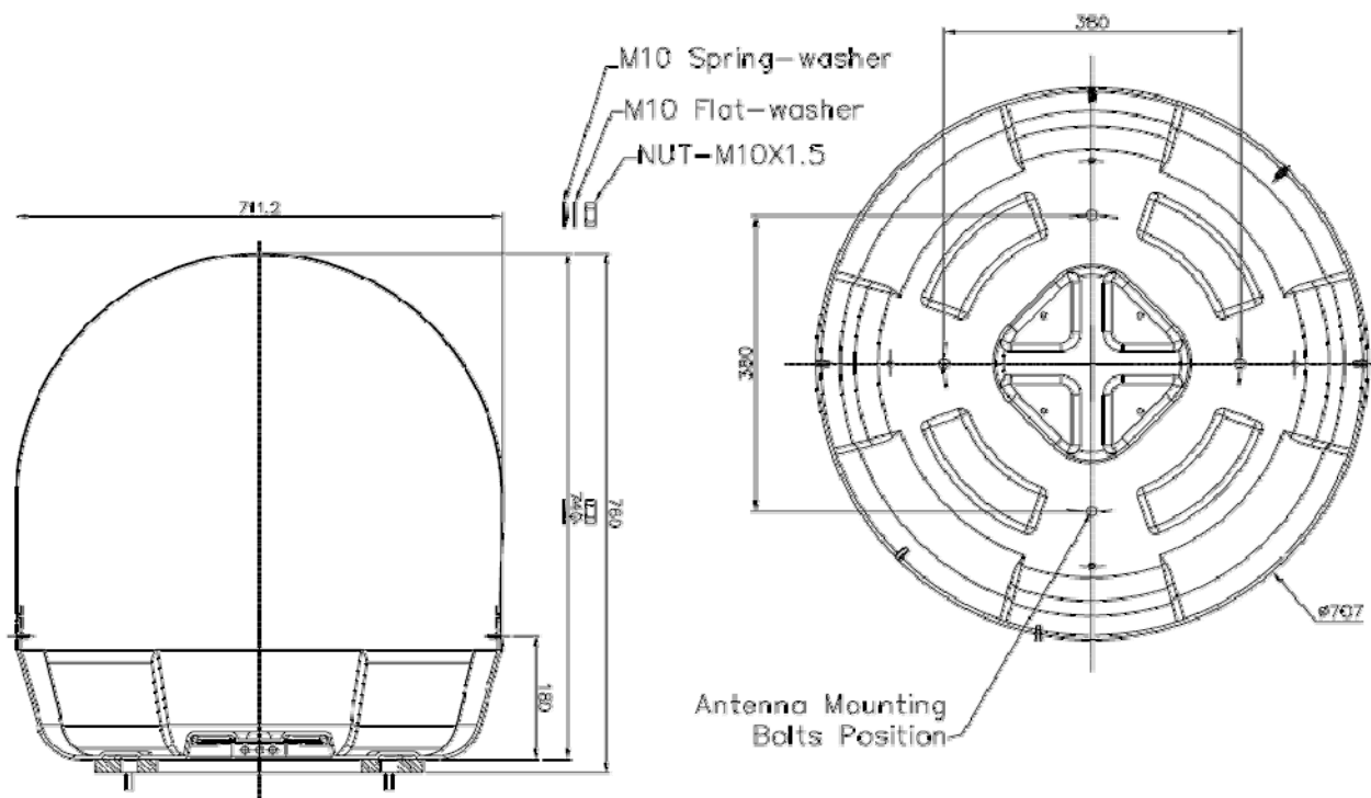
Figure D-4 Schéma de l'antenne Ocean Line 360/460
