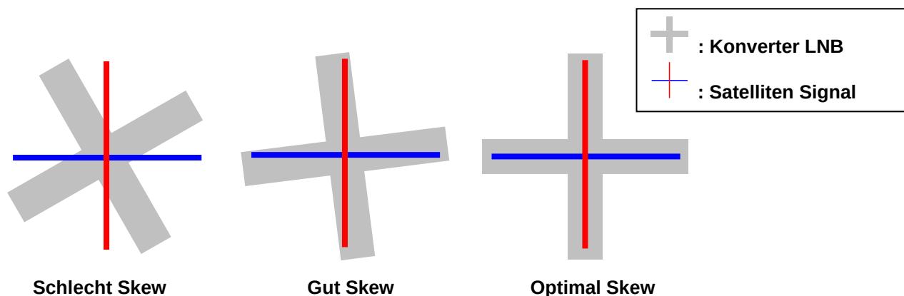
Abb. 2-4 Besten Skew-Winkel
