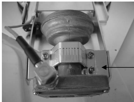
Abb. A-4 LNB des Free Way-Antennen
