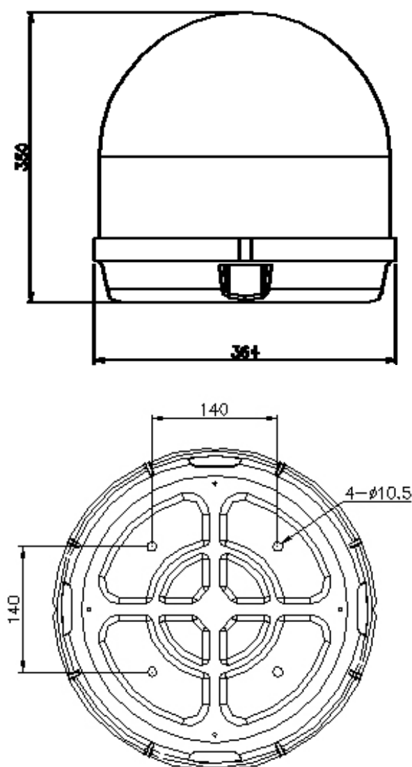
Figura D-1 Disegni dell'antenna Ocean Line 132
