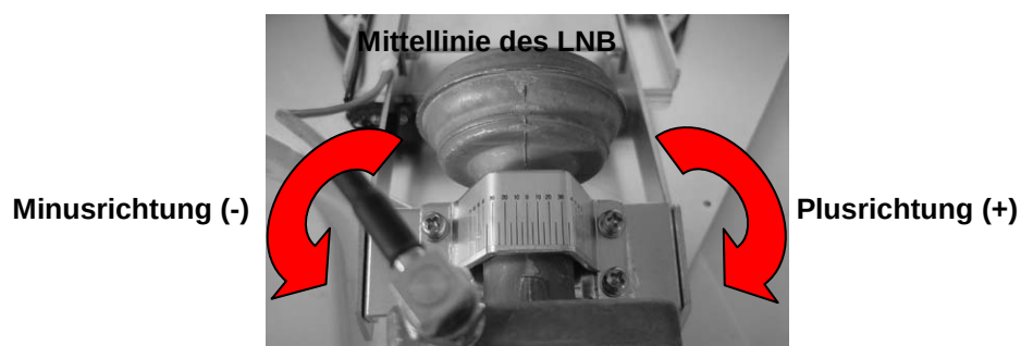
Abb. A-5 Einstellung des Skew-Winkels (LNB-Tilt) Free Way
